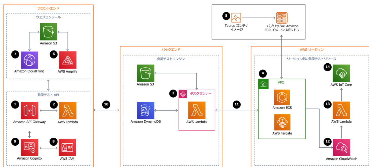
AWS での分散負荷テストソリューションのアーキテクチャ
