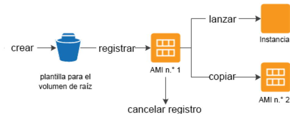
Figura 3: Uso de una AMI para lanzar y realizar una copia de seguridad de una instancia
