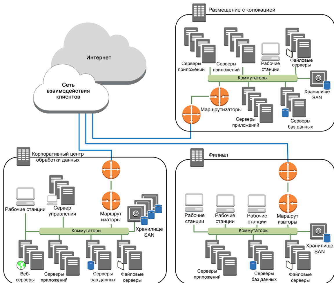
Рис. 5. Локальная среда
